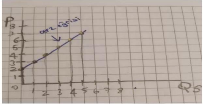
Şekil 2.3. Arz eğrisi ( Q_s = -2 + P arz fonksiyonu için)
